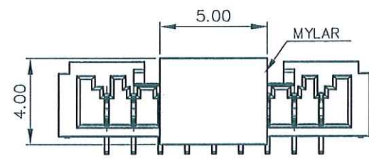
△3809K-XXXM-XOX: ADD MYLAR
